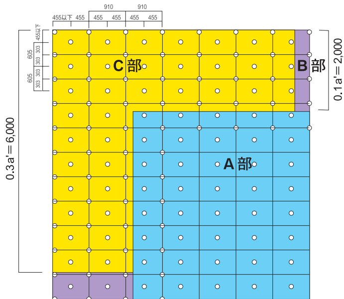
[標準固定ピッチ図例および安全率]
