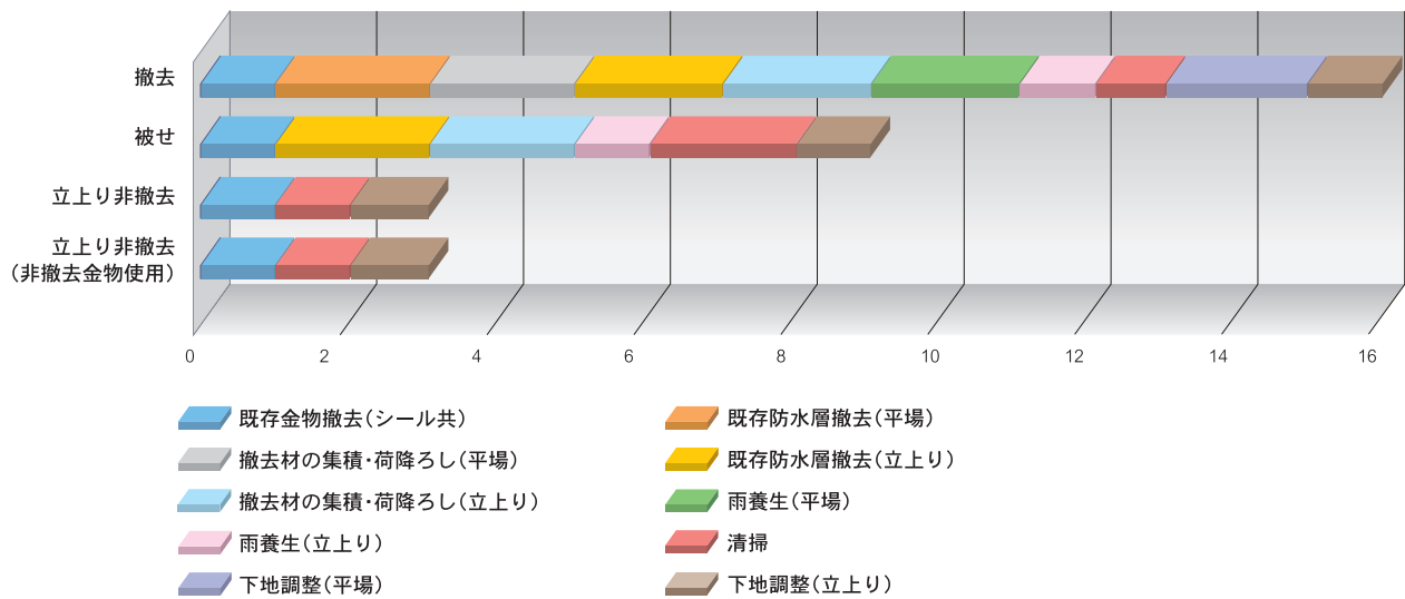
各工法の防水層新設までの作業工程比較表
