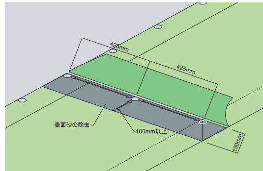
■ 短辺接合部の処理方法
