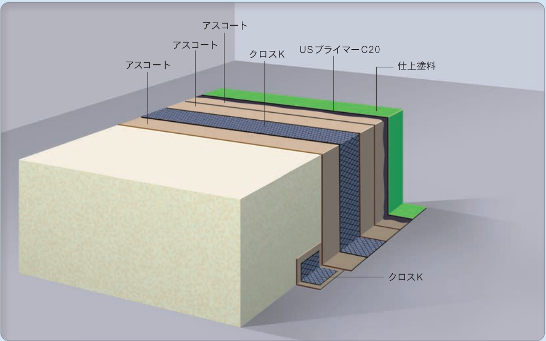
架 台 回 り
