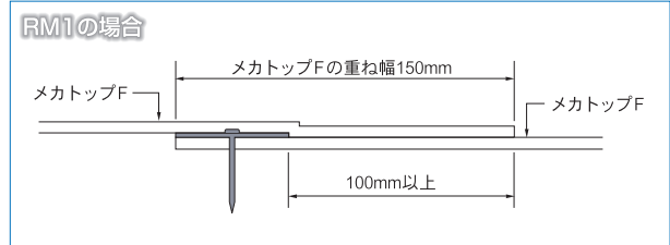
■ メカディスクC 打込み位置
