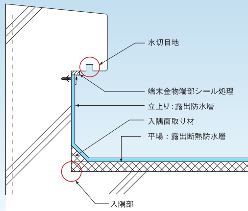
▲露出アスファルト防水
